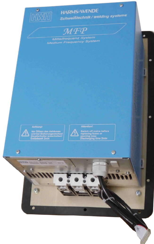
Abb. 5-1 MFP -Leistungsteil
